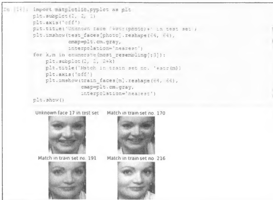
Рис. 14.3. Вывод демонстрирует результаты, которые напоминают тестовое изображение
