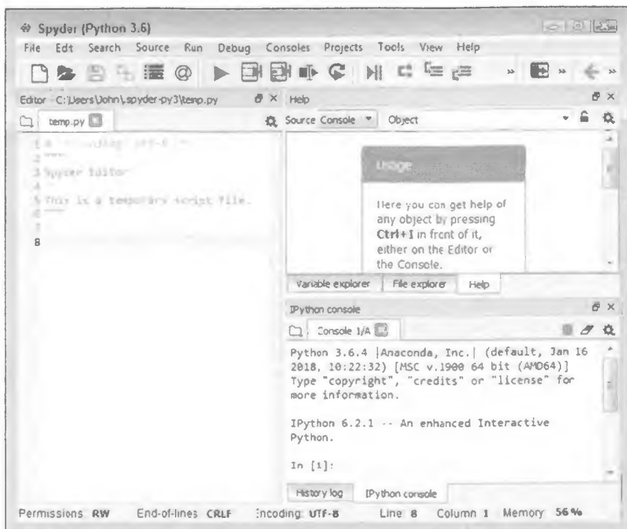
Рис. 2.5. IDE Spyder
