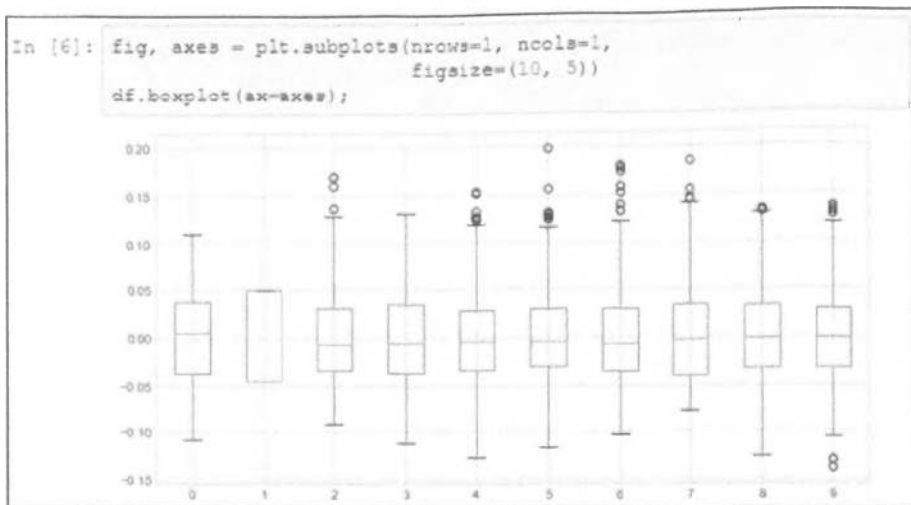
Рис. 16.2. Диаграмма размаха
