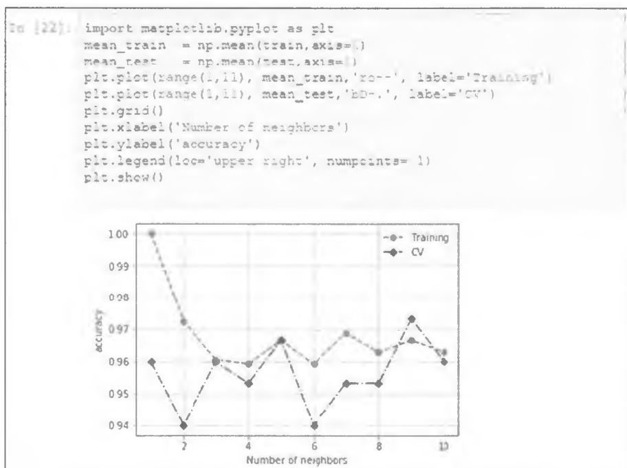
Рис. 18.2. Кривые проверки
