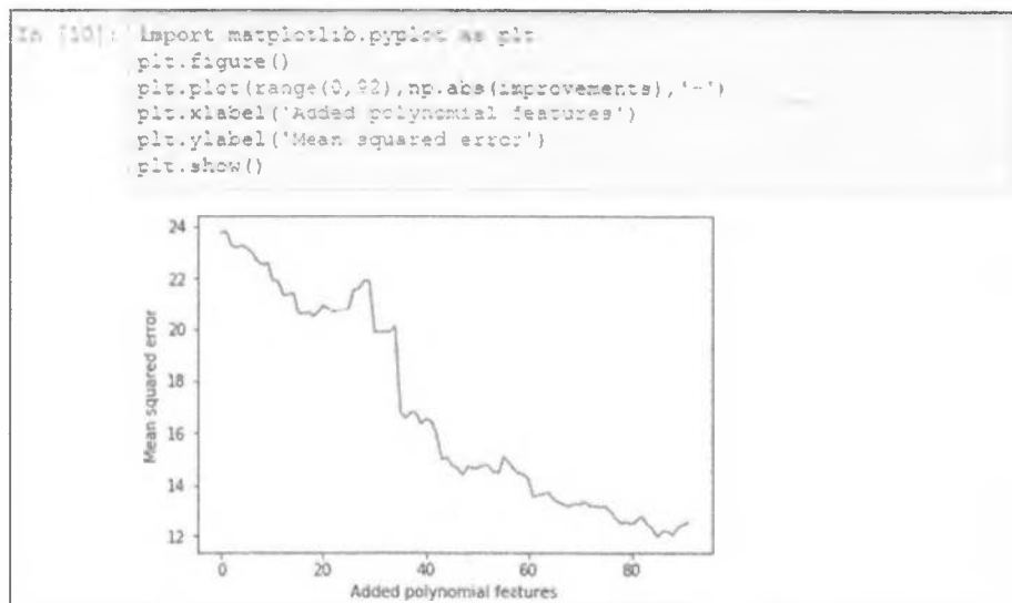
Рис. 19.3. Добавление полиномиальных функций увеличивает силу прогнозирования
