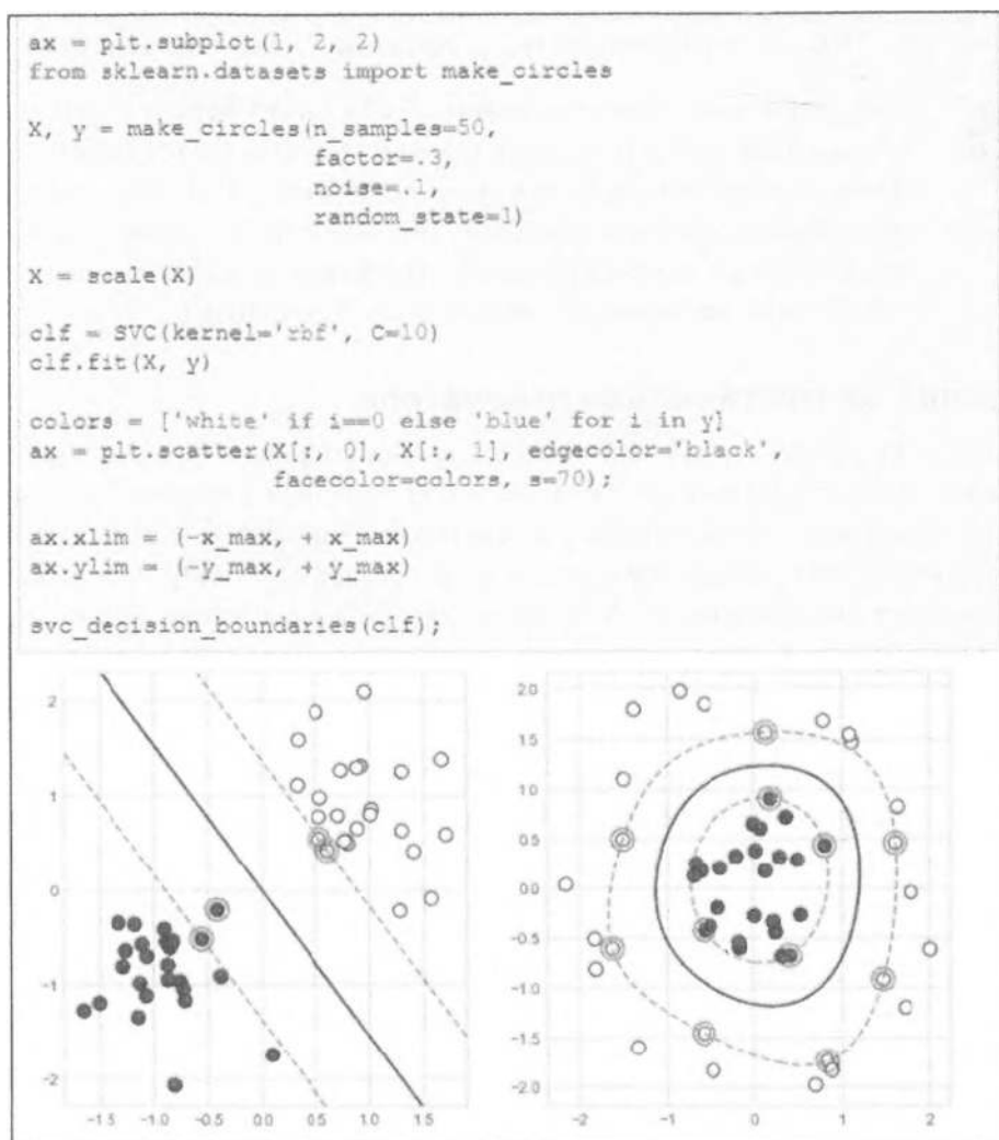
Рис. 19.6. Подходящее решение SVM для задачи двух и более групп
