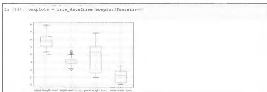
Рис. 13.4. Диаграмма размаха, упорядоченная по переменным
