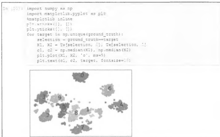
Рис. 14.1. Результирующая проекция набора данных рукописных цифр по алгоритму t-SNE
